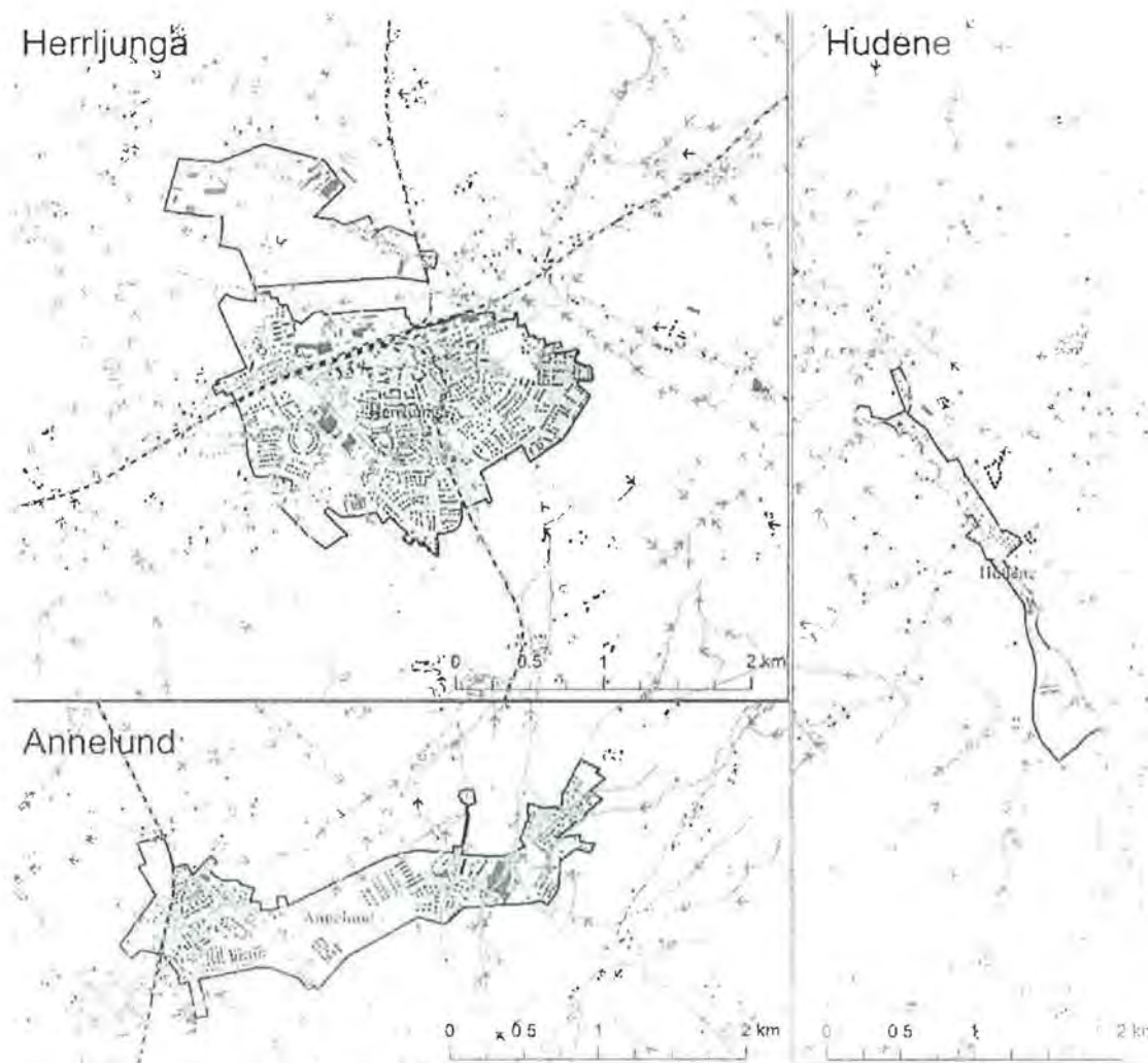
Figur 10 Översvämningsanalys. Avrinning på markytan redovisas med blå linjer och pilar. Låglanta områden med översvämningsrisk är gråskrafferade
